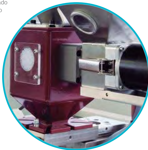
Moldagem de acessórios por injeção Extrusão de perfis
